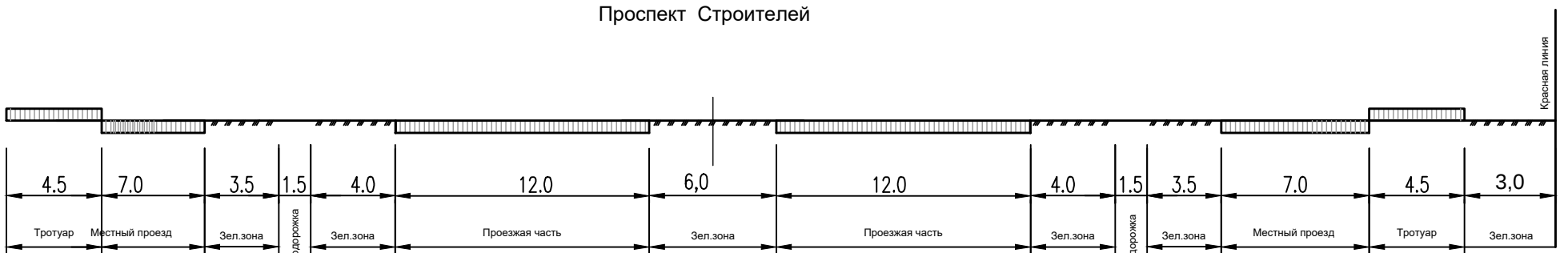
Поперечные профили автомобильных дорог вокруг микрорайона № 7
